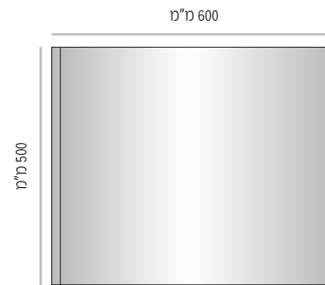
LVD-P-600-500 מק"ט 500 מ"מ גובה מידת אינסרט 500 מ"מ x 584 מ"מ
