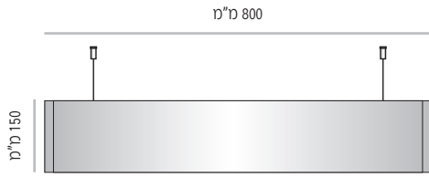
LVD-DS-P-800-150 מק"ט 150 מ"מ גובה 150 מ"מ x 785 מ"מ מידת אינסרט
